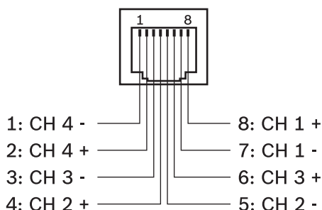
Obrázek 6.1: Obsazení vývodů u zásuvky LINE IN 1-4
