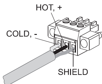
Obrázek 6.2: Symetrické kabely
