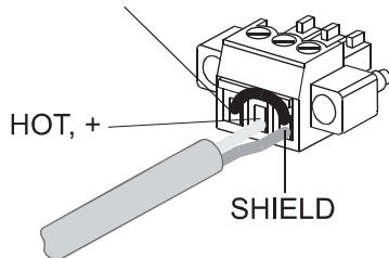
Obrázek 6.3: Nesymetrické kabely
